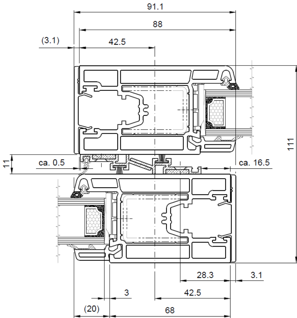
Creon schuifpui zonder aanslag, EvolutionDrive SF, tussendetail
